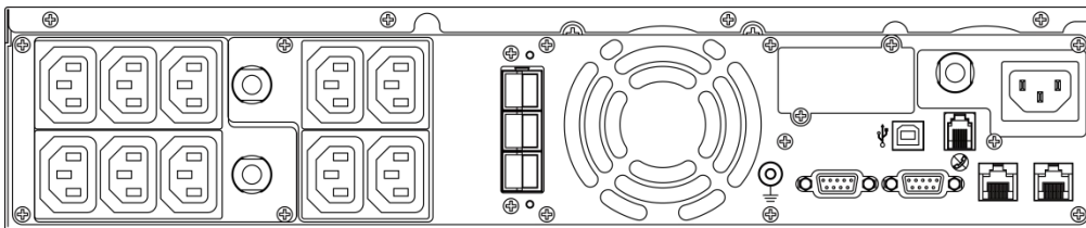
Face Arrière Elite PRO 1000ELCDRTXL2U Elite PRO 1500ELCDRTXL2U
